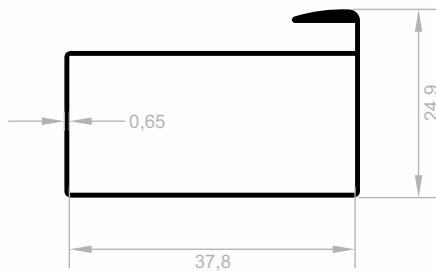
J 8575 SPECIAL PROFILES WEIGHT : 0,243 kg/m
