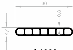
J 1068 SPECIAL PROFILES WEIGHT : 0,173 kg/m
