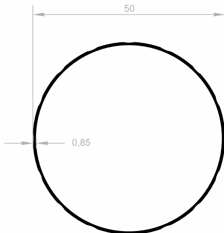
J 1093 SPECIAL PROFILES WEIGHT : 0,339 kg/m
