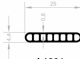
J 1201 SPECIAL PROFILES WEIGHT : 0,162 kg/m
