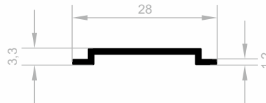
J 1130 SPECIAL PROFILES WEIGHT : 0,111 kg/m
