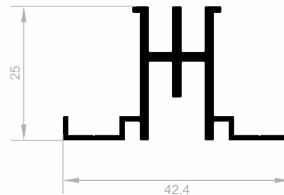
J 3336 SPECIAL PROFILES WEIGHT : 0,480 kg/m
