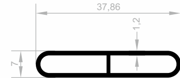
J 1032 SPECIAL PROFILES WEIGHT : 0,273 kg/m
