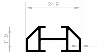
J 3356 SPECIAL PROFILES WEIGHT : 0,220 kg/m
