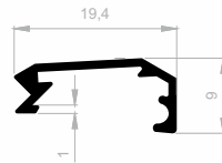
J 1180 DISPLAY PROFILE WEIGHT : 0,108 kg/m
