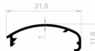
J 1182 DISPLAY PROFILE WEIGHT : 0,138 kg/m
