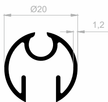
J 1188 DISPLAY PROFILE WEIGHT : 0,247 kg/m
