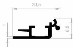
J 1184 DISPLAY PROFILE WEIGHT : 0,121 kg/m
