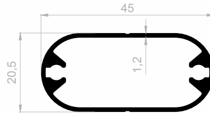
J 1056 DISPLAY PROFILE WEIGHT : 0,490 kg/m
