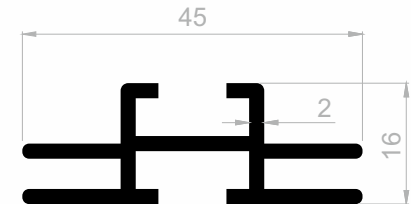
J 1186 DISPLAY PROFILE WEIGHT : 0,594 kg/m
