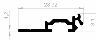
J 19120 DISPLAY PROFILE WEIGHT : 0,146 kg/m
