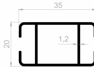
J 1185 DISPLAY PROFILE WEIGHT : 0,405 kg/m
