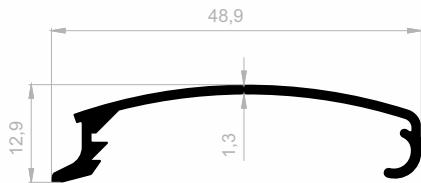
J 1181 DISPLAY PROFILE WEIGHT : 0,275 kg/m
