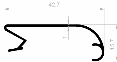
J 1160 DISPLAY PROFILE WEIGHT : 0,217 kg/m
