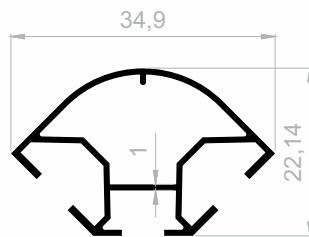
J 1963 DISPLAY PROFILE WEIGHT : 0,287 kg/m
