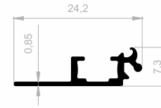
J 8215 DISPLAY PROFILE WEIGHT : 0,111 kg/m
