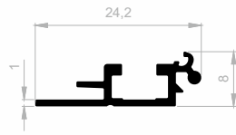
J 1988 DISPLAY PROFILE WEIGHT : 0,138 kg/m
