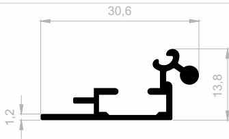
J 1163 DISPLAY PROFILE WEIGHT : 0,228 kg/m
