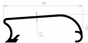
J 1183 DISPLAY PROFILE WEIGHT : 0,273 kg/m
