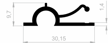
J 1173 DISPLAY PROFILE WEIGHT : 0,205 kg/m
