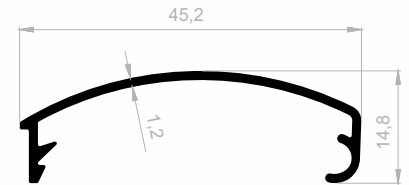
J 1579 DISPLAY PROFILE WEIGHT : 0,233 kg/m
