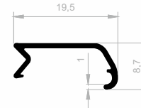
J 1199 DISPLAY PROFILE WEIGHT : 0,089 kg/m
