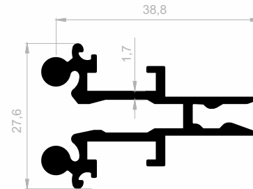
J 1162 DISPLAY PROFILE WEIGHT : 0,688 kg/m
