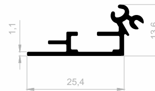
J 19123 DISPLAY PROFILE WEIGHT : 0,222 kg/m
