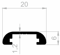
J 1509 DISPLAY PROFILE WEIGHT : 0,140 kg/m
