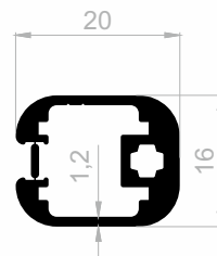
J 1510 DISPLAY PROFILE WEIGHT : 0,352 kg/m
