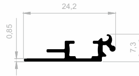
J 19126 DISPLAY PROFILE WEIGHT : 0,122 kg/m
