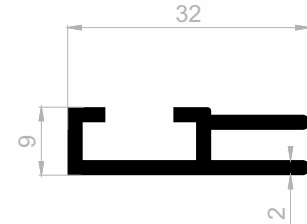
J 1187 DISPLAY PROFILE WEIGHT : 0,348 kg/m
