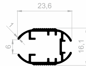
J 1613 DISPLAY PROFILE WEIGHT : 0,245 kg/m
