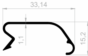
J 19125 DISPLAY PROFILE WEIGHT : 0,157 kg/m
