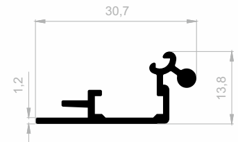
J 1179 DISPLAY PROFILE WEIGHT : 0,224 kg/m
