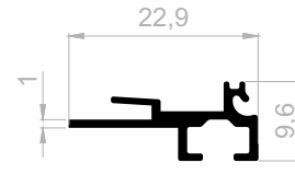
J 1162 DISPLAY PROFILE WEIGHT : 0,688 kg/m
