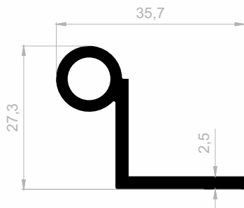
J 1943 HINGE PROFILES WEIGHT : 0,477 kg/m
