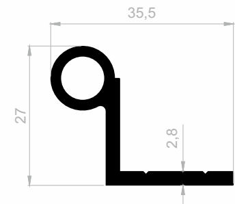
J 1141 HINGE PROFILES WEIGHT : 0,494 kg/m
