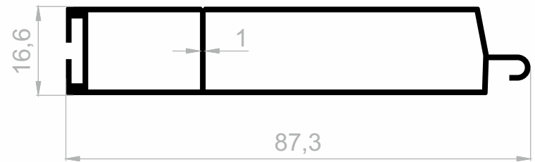
J 6042 ROLLER SHUTTERS WEIGHT : 0,658 kg/m
